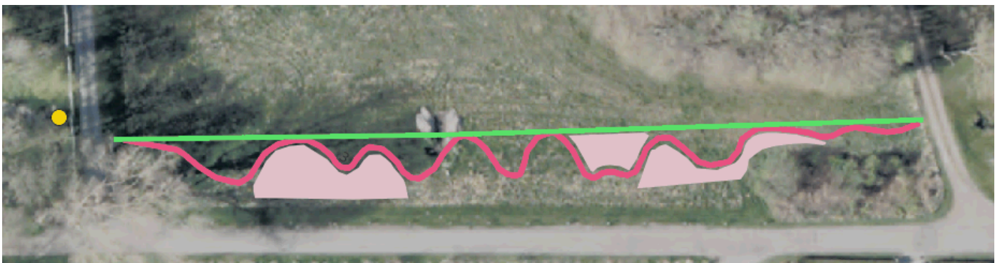
Figur 1 Gadholt bæks nuværende forløb (grøn streg) samt projektforslag (lyserød streg). Brinkerne vil være fladere i de lyserøde områder. Indløb under rørbro til Hullvej 8 er markeret med gul.
