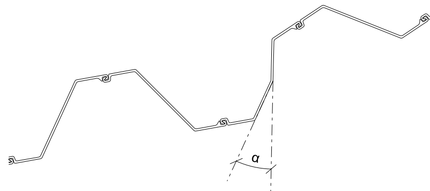
DETALJE MED EKSEMPEL FOR BUKKET SPUNSJERN, 1:25
