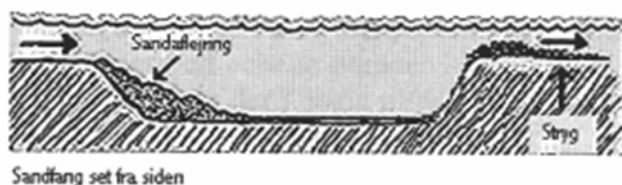
Principtegning af sandfang
