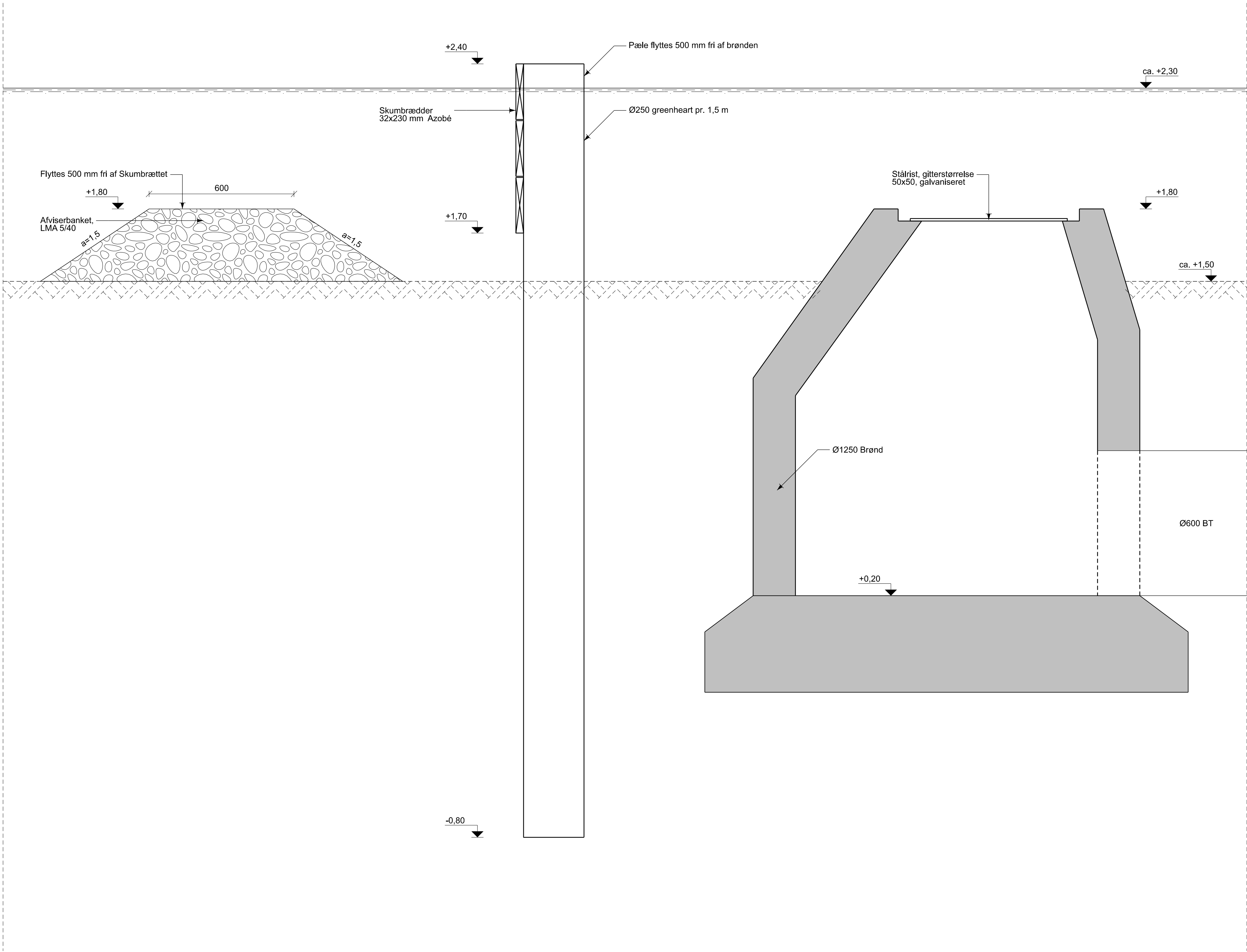
AFVISERBANKET OG INDLØBSBYGVÆRK 1:10
