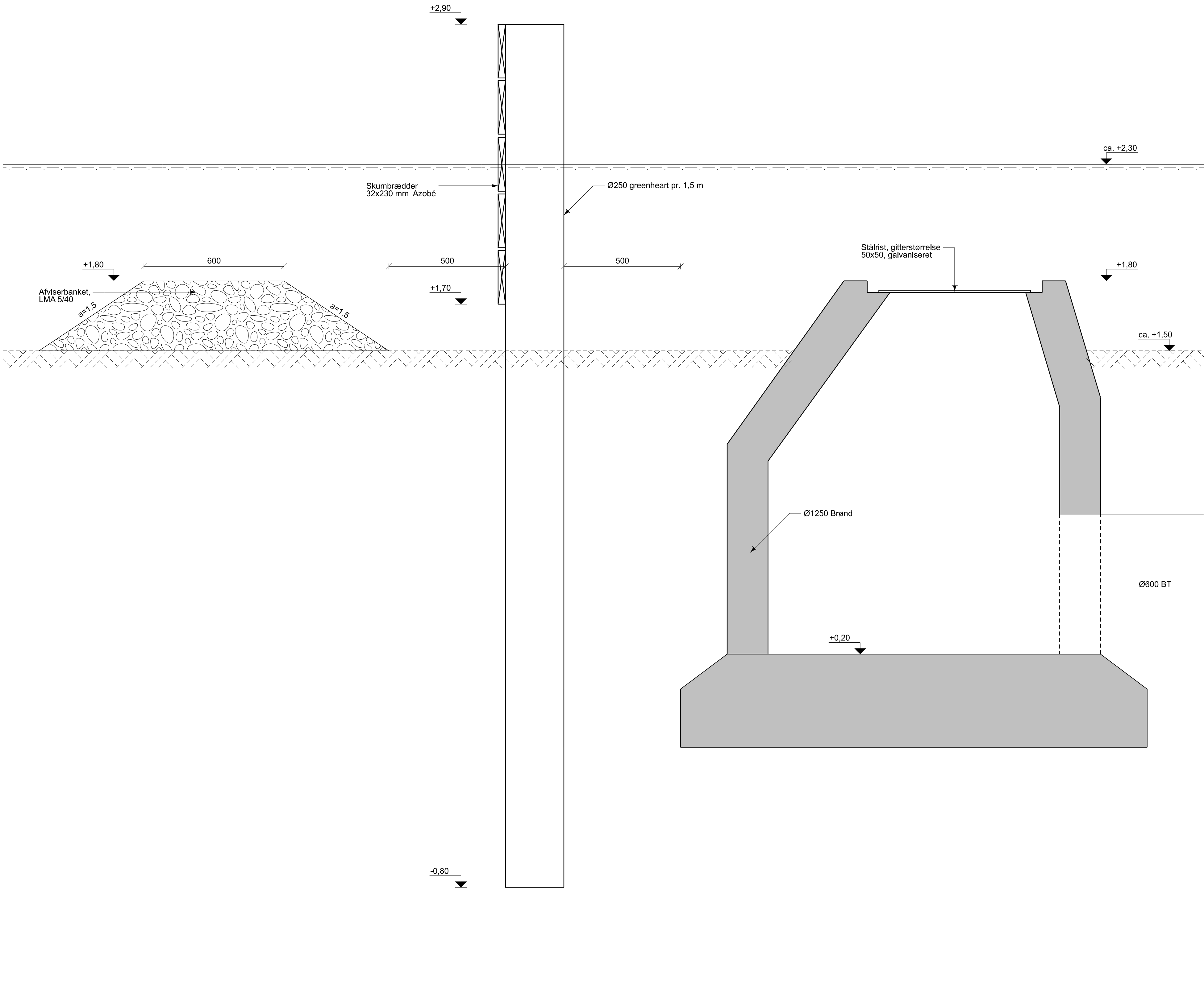
AFVISERBANKET OG INDLØBSBYGVÆRK 1:10
