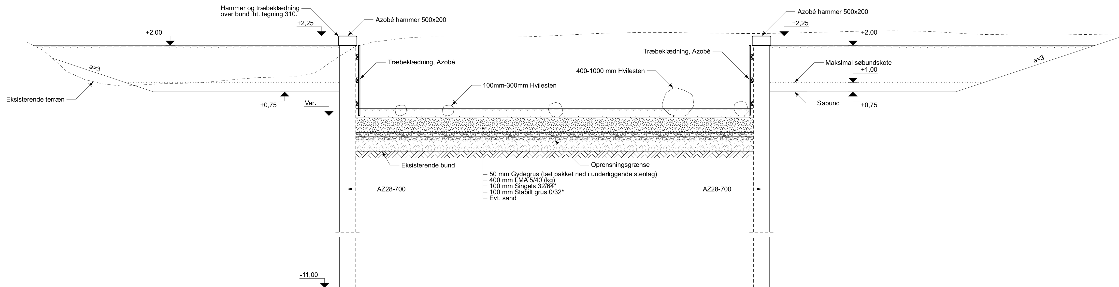
TVÆRSNIT C-C, 1:50
